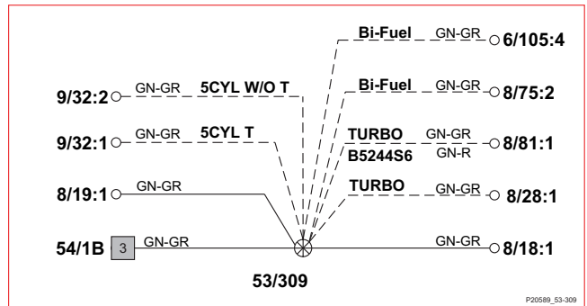
53/309 8 缸
