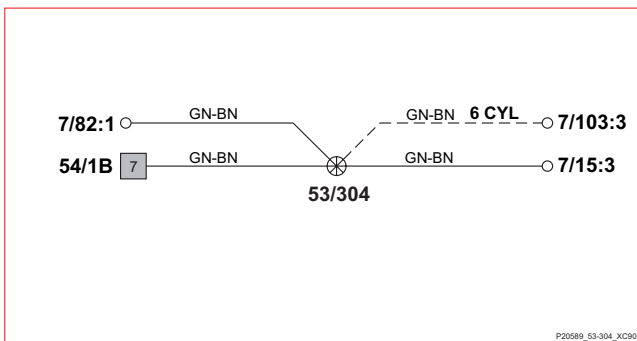
53/304 5 缸帶渦輪 / 6 缸
