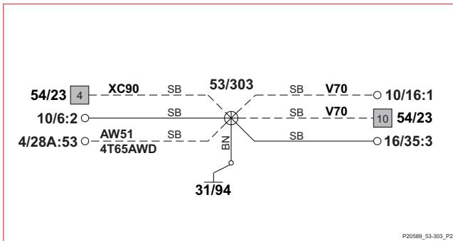
53/304 5 缸不帶渦輪
